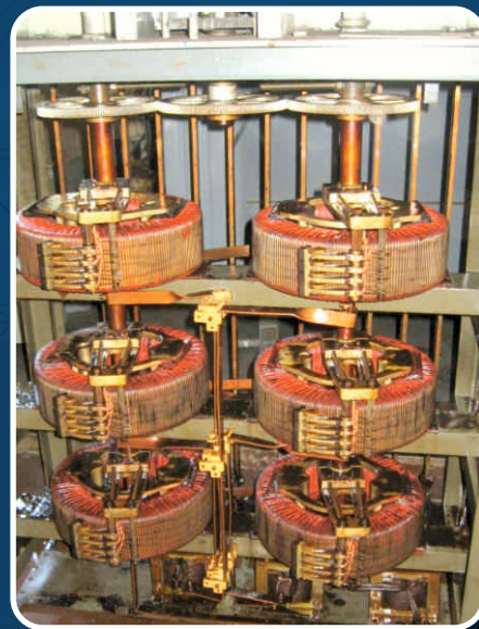
DIMMERSTAT 400 AMP
